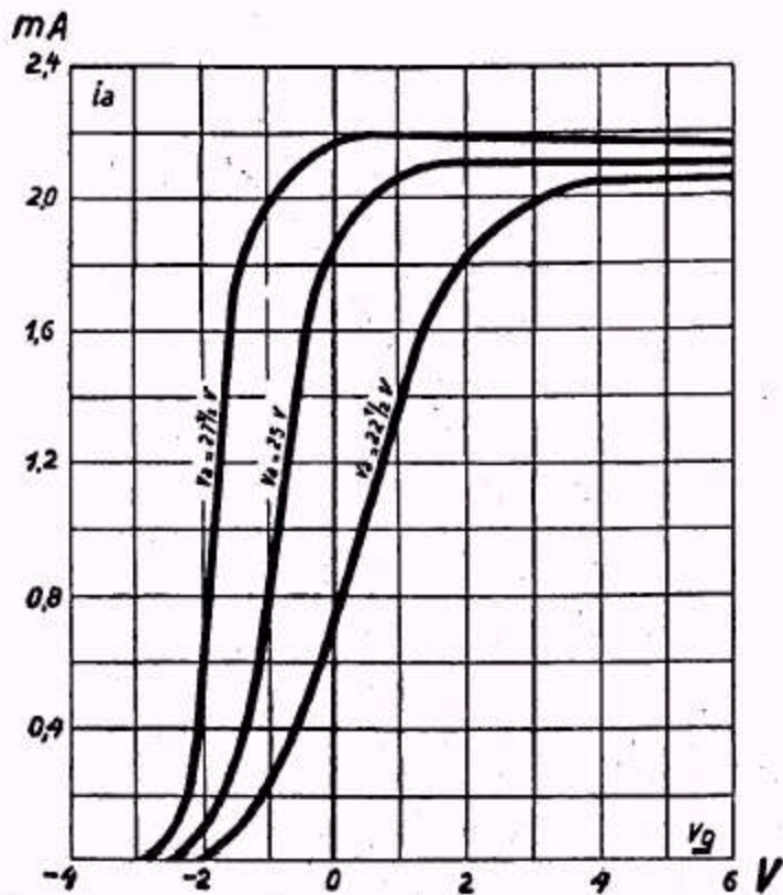
Abb. 149. Kennlinien der Philips-Thoriumröhre B II. (Anhang Nr. 56).
